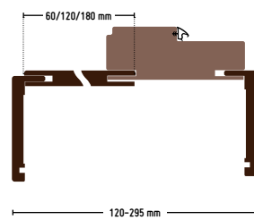
Allargamento Добор Frame extension Élargissement
